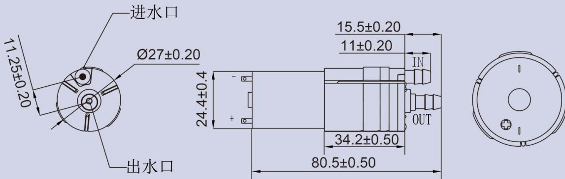
產品構造圖 Dimension Drawing
