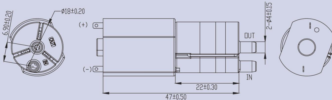
產品構造圖 Dimension Drawing
