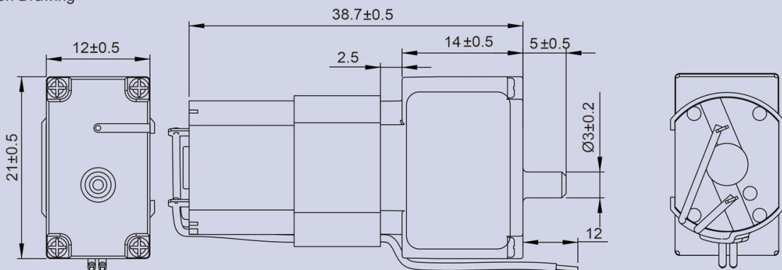
產品構造圖 Dimension Drawing
