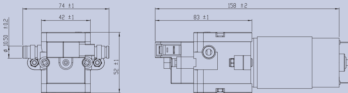
產品構造圖 Dimension Drawing
