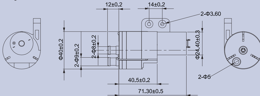
產品構造圖 Dimension Drawing
