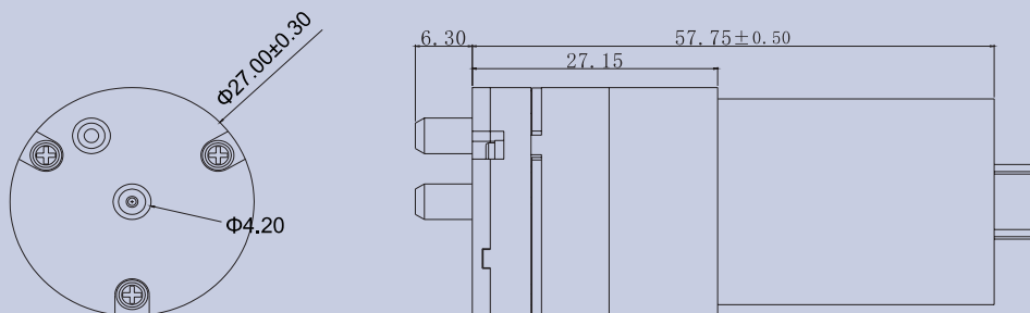
產品構造圖 Dimension Drawing
