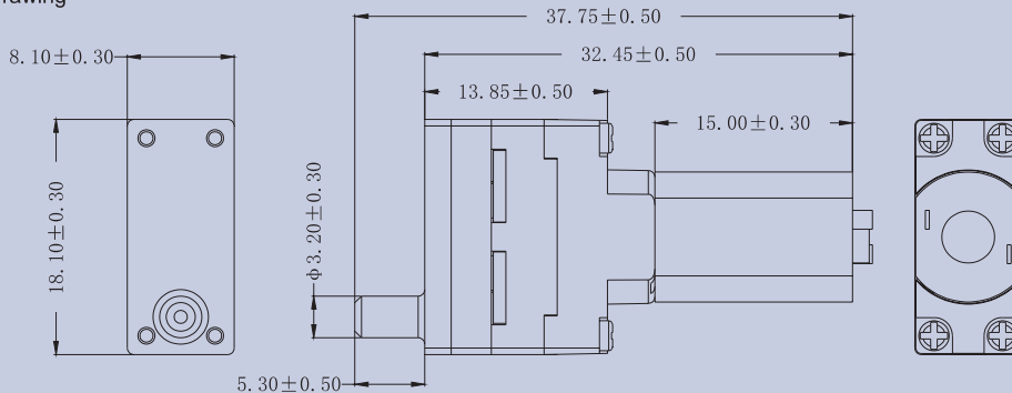
產品構造圖 Dimension Drawing
